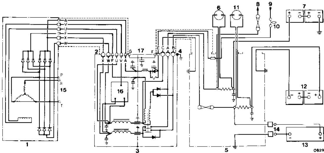
Fig. 151 Charging circuit—24 volt 90 amp
